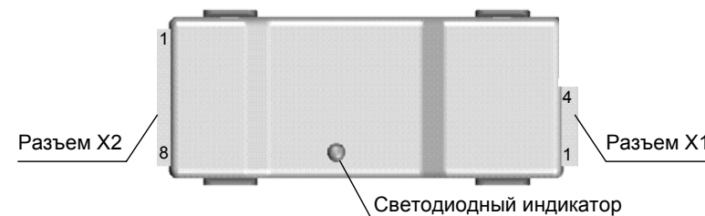
Рисунок 1. Внешний вид и расположение разъемов адаптера.
