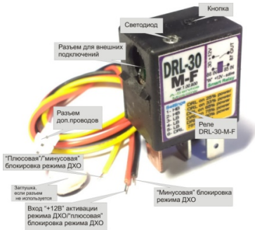
Рис 4. Внешний вид реле-контроллера DRL-30-M-F
