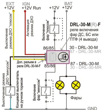
Рис. 2. «Полное подключение» DRL-30-M(MR)-F для управления фарами ДС, БС или ПТФ с обеспечением «Режима ДХО».
