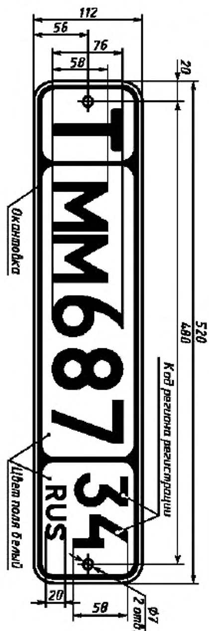
Рисунок А.19 — Регистрационный знак типа 19
